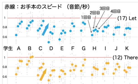
図1：学生の発話スピード（音節/秒）の上達
