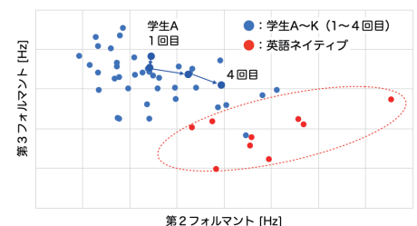
図3：学生全体と英語ネイティブの分布差
